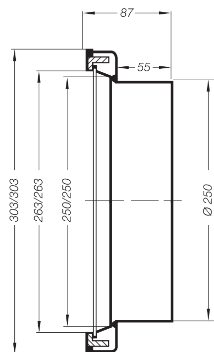
Einbaudose Typ 358
